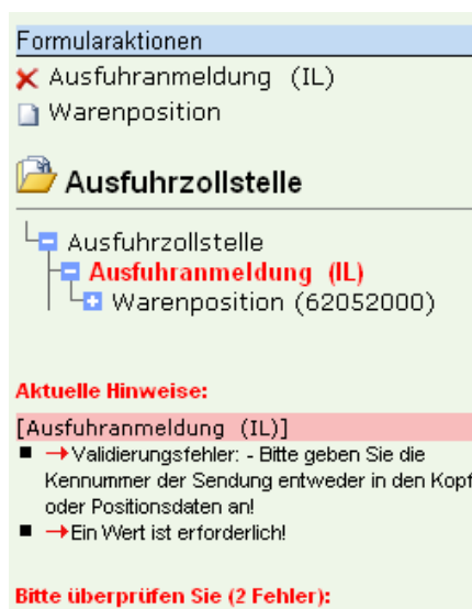
Abbildung: Hinweis-/Prüfenster
