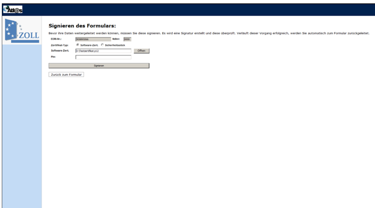
Abbildung: Signieren
