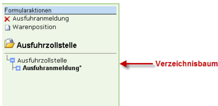
Abbildung: Verzeichnisbaum
